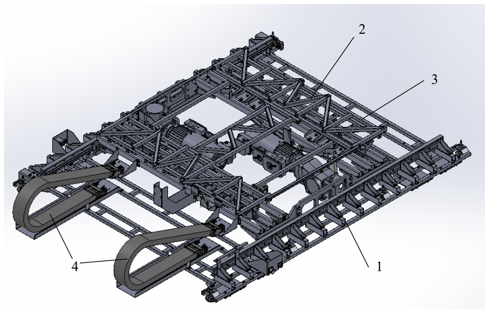
Рисунок 8 – Динамическая платформа
