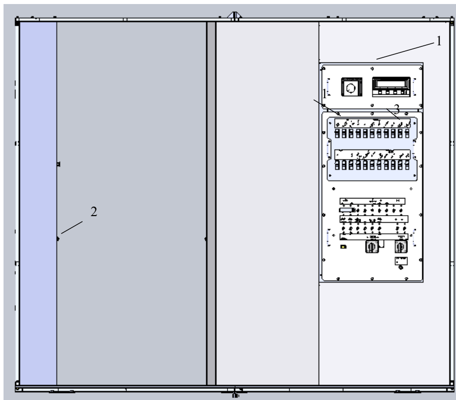
Рисунок 7 – Оборудование кабины (задняя часть)
