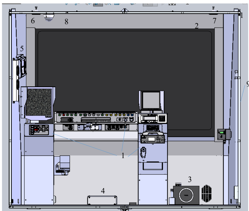
Рисунок 6: Оборудование кабины (передняя часть)
